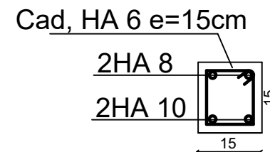
LINTEAU (15x15)
