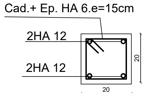
Poutre noyée PN (20x20)
