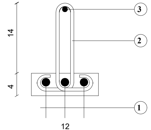
Schéma nervure
